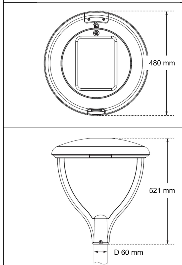
Rozměry - uchycení
