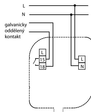
4 - vodičové zapojení
